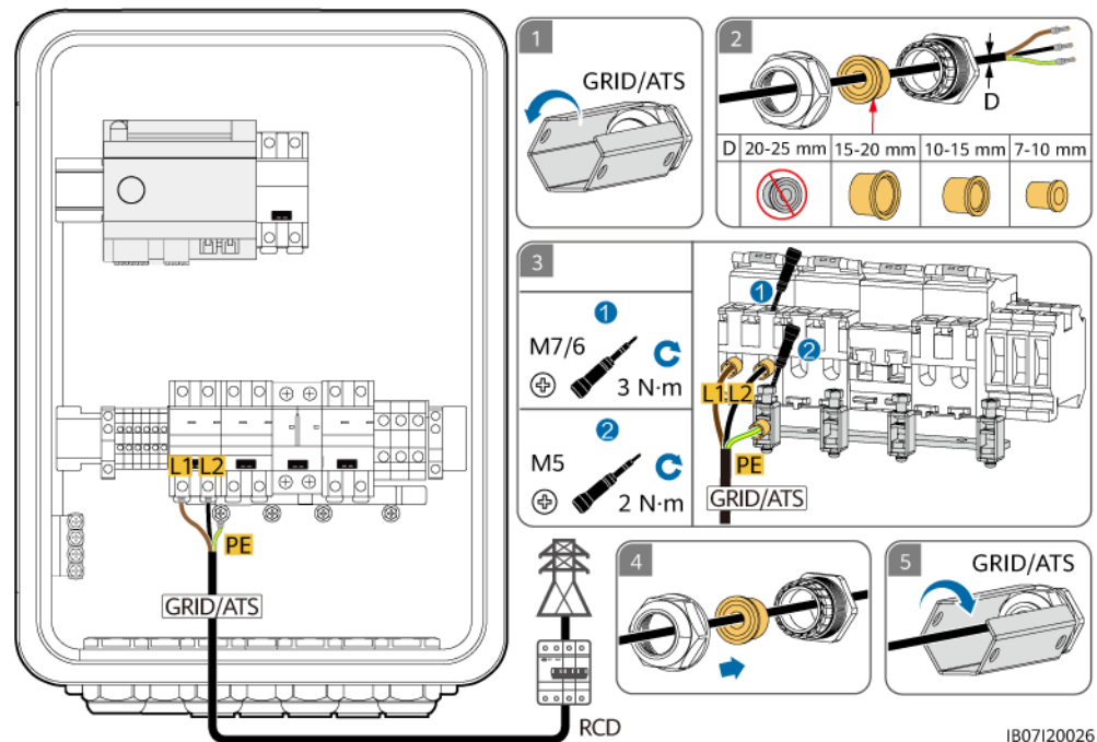
Abbildung 5-12 Anschließen des Netz-AC-Ausgangsstromkabels (L1/L2 Dual-Live-Kabelverbindung)
