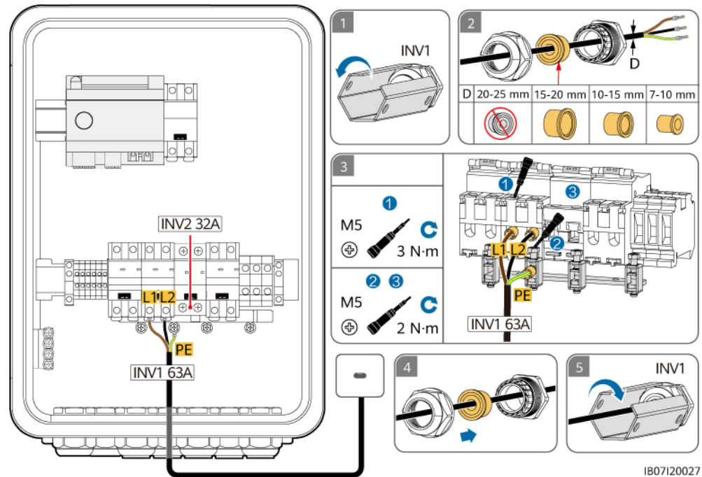
Abbildung 5-16 Anschließen des AC-Eingangskabels vom Wechselrichter (L1/L2 Dual-Live-Kabelverbindung)
