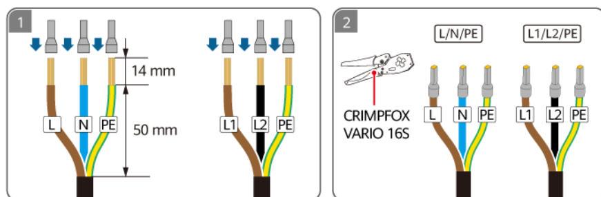
Abbildung 5-17 Crimpen der AC-Kabelendverschlüsse des SmartGuard-63A-S0
