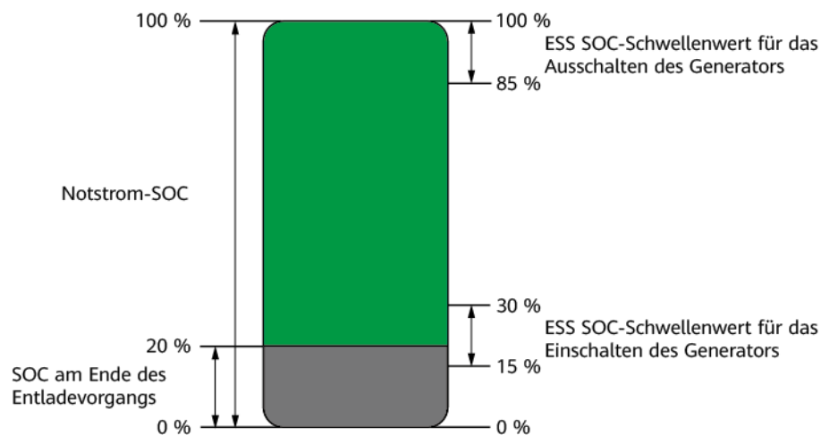
Abbildung 6-12 Batterie-SOC
