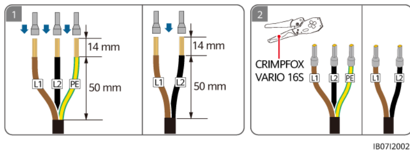
Abbildung 5-10 Crimpen der AC-Kabelndklemmen (L1/L2 Dual-Live-Kabelverbindung)
