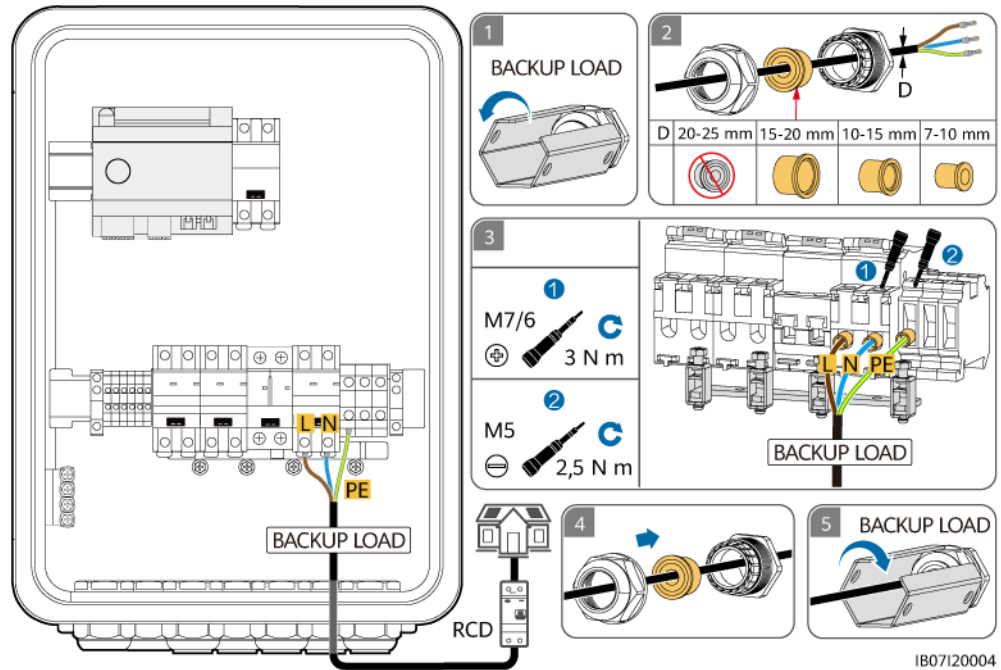
Abbildung 5-19 Anschließen des Ausgangsstromkabels der Backup-Last der SmartGuard-63A-S0
