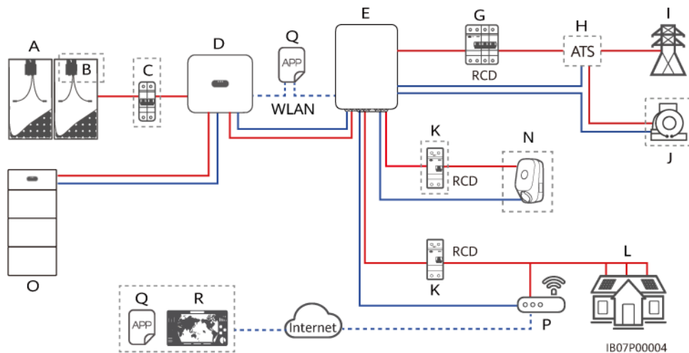
Abbildung 2-4 Vernetzung aller Lasten, die an die SmartGuard angeschlossen sind (gestrichelte Kästchen weisen auf optionale Komponenten hin)
