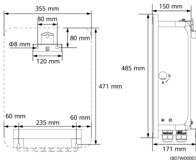
Abbildung 4-1 Abmessungen der Montagehalterung
