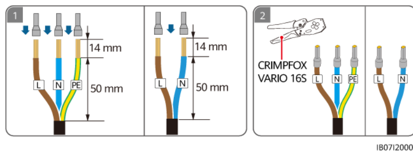
Abbildung 5-21 Crimpen der AC-Kabelendklemmen (L/N Single-Live-Kabelverbindung)
