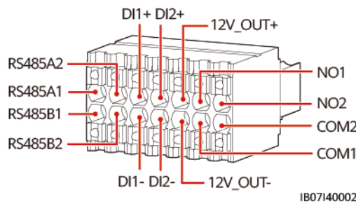
Abbildung 5-28 Definition der Pins
