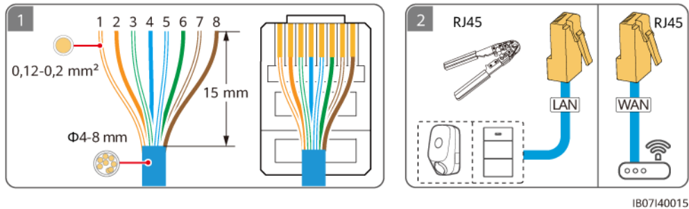
Abbildung 5-31 FE-Kommunikationskabel (gestrichelte Kästchen weisen auf optionale Komponenten hin)
