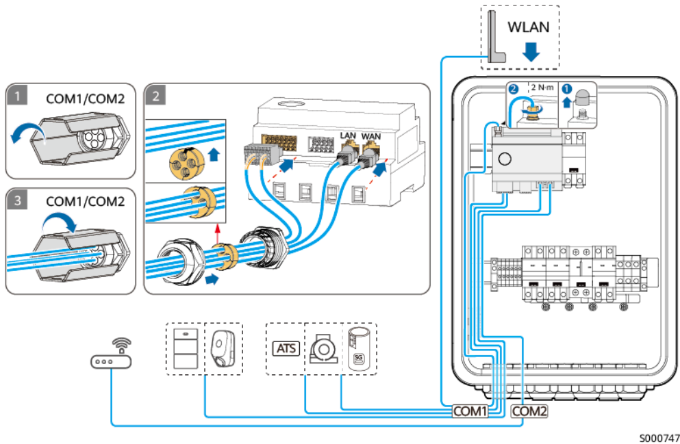
Abbildung 5-32 Anschluss von SmartAssistant-Signalkabeln (gestrichelte Kästchen weisen auf optionale Komponenten hin)
