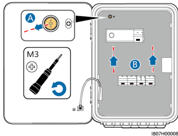
Abbildung 5-6 Öffnen des Deckels des Wartungsfachs
