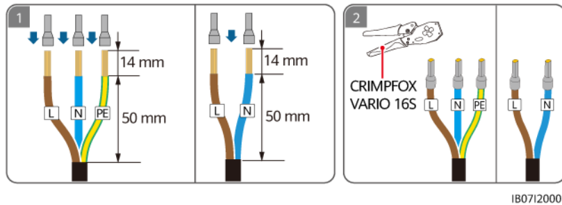
Abbildung 5-9 Crimpen der AC-Kabelndklemmen (L/N Single-Live-Kabelverbindung)
