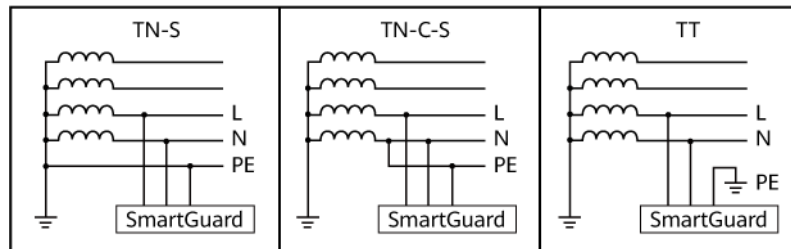
Abbildung 2-7 Erdungssystem (L/N Single-Live-Kabelverbindung)
