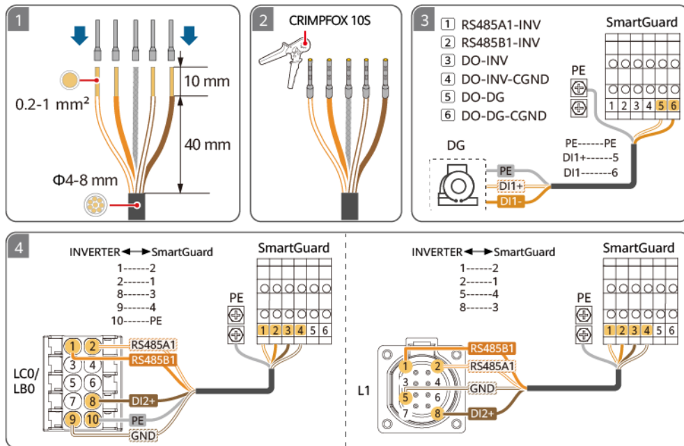
Abbildung 5-25 Crimpen der Kabelendverschlüsse des Signalkabels (das gestrichelte Kästchen zeigt eine optionale Komponente an)
