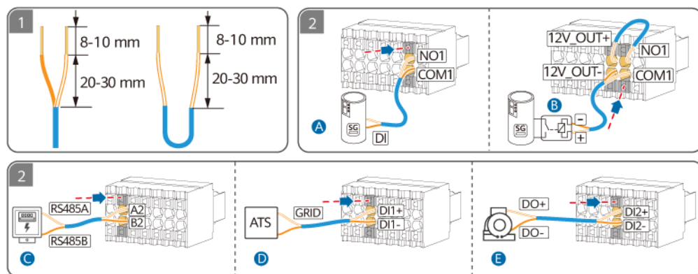
Abbildung 5-29 Anschluss des Signalkabels an die 14-polige Klemme
