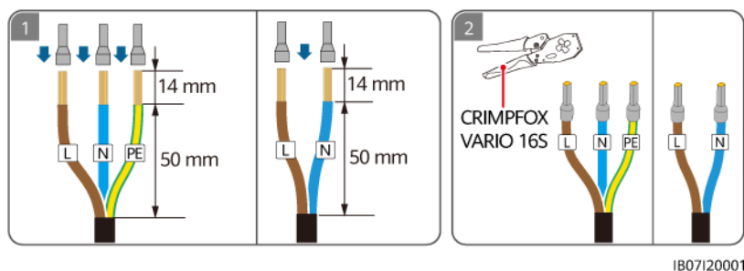
Abbildung 5-13 Crimpen der AC-Kabelendklemmen (L/N Single-Live-Kabelverbindung)
