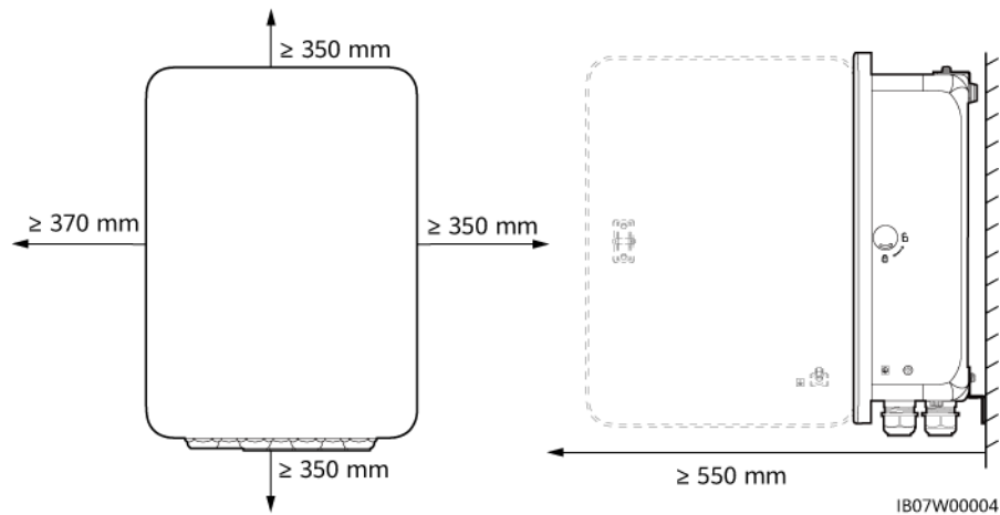
Abbildung 4-2 Abstände
