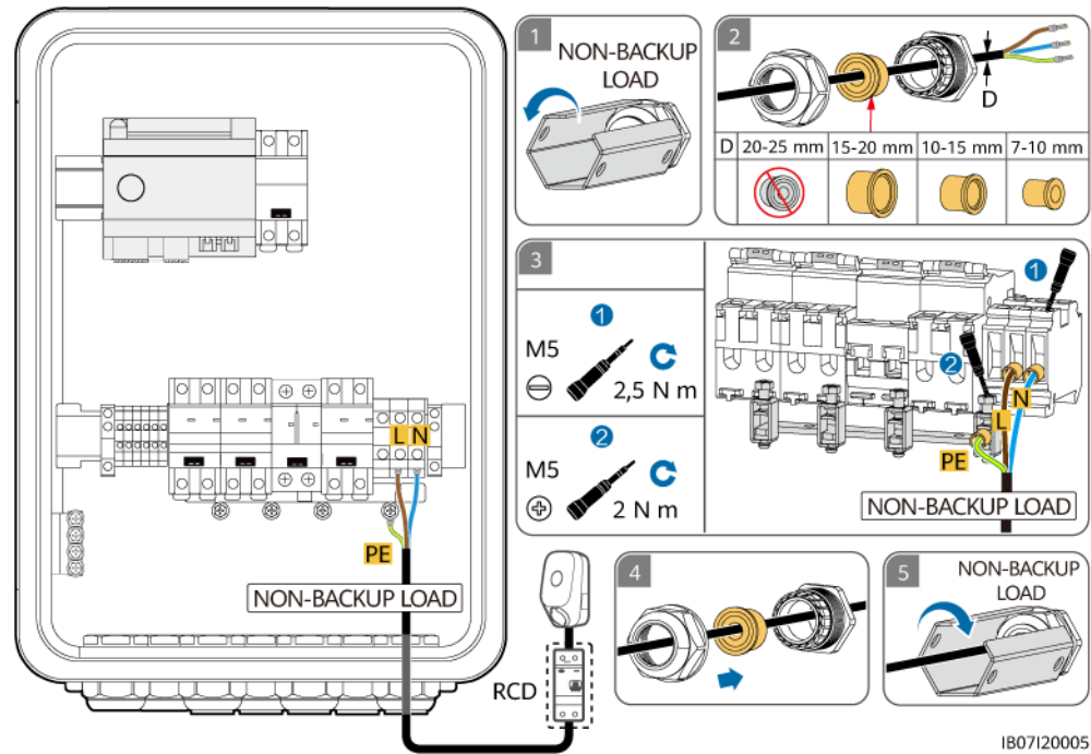
Abbildung 5-23 Anschließen des Ausgangsstromkabels der Nicht-Backup-Last (L/N Single-Live-Kabelverbindung)
