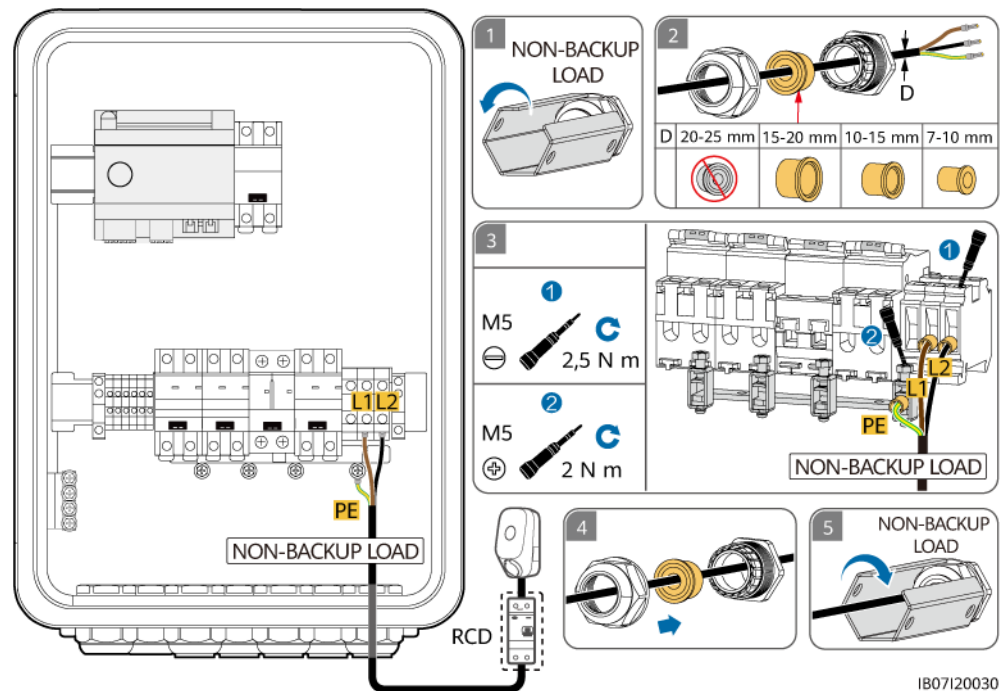
Abbildung 5-24 Anschließen des Ausgangsstromkabels der Nicht-Backup-Last (L1/L2 Dual-Live-Kabelverbindung)
