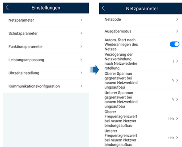
Abbildung 6-8 Einstellen des Ausgangsmodus
