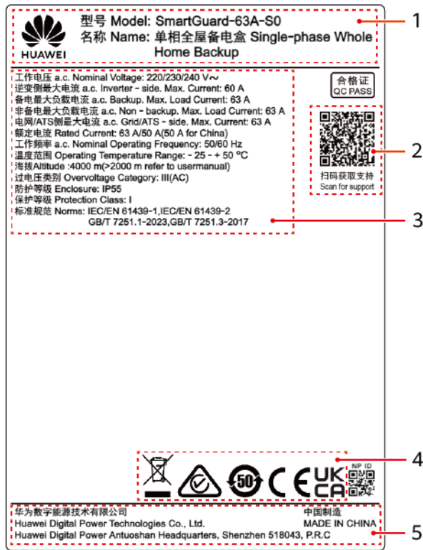
Abbildung 2-13 Typenschild (am Beispiel von SmartGuard-63A-S0)
