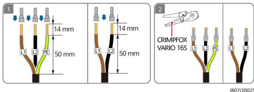
Abbildung 5-14 Crimpen der AC-Kabelendklemmen (L1/L2 Dual-Live-Kabelverbindung)
