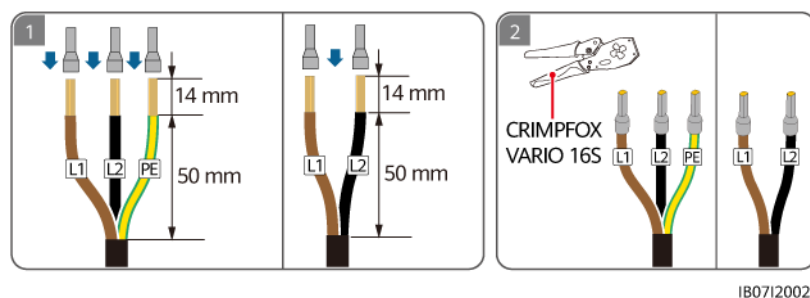
Abbildung 5-22 Crimpen der AC-Kabelendklemmen (L1/L2 Dual-Live-Kabelverbindung)
