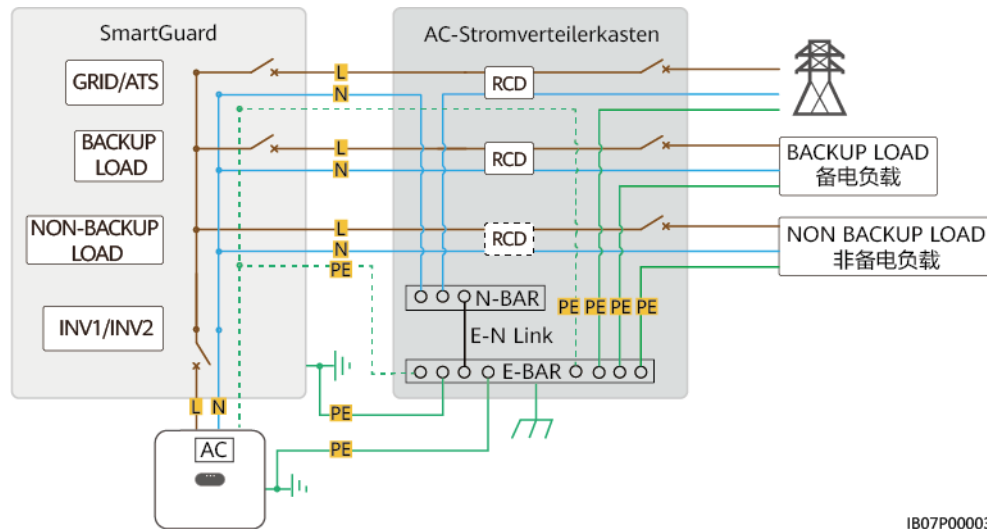
Abbildung 2-3 SmartGuard-63A-AUS0 Schaltplan für Wohngebäude (gestrichelte Linien stehen für optionale Kabelanschlüsse)
