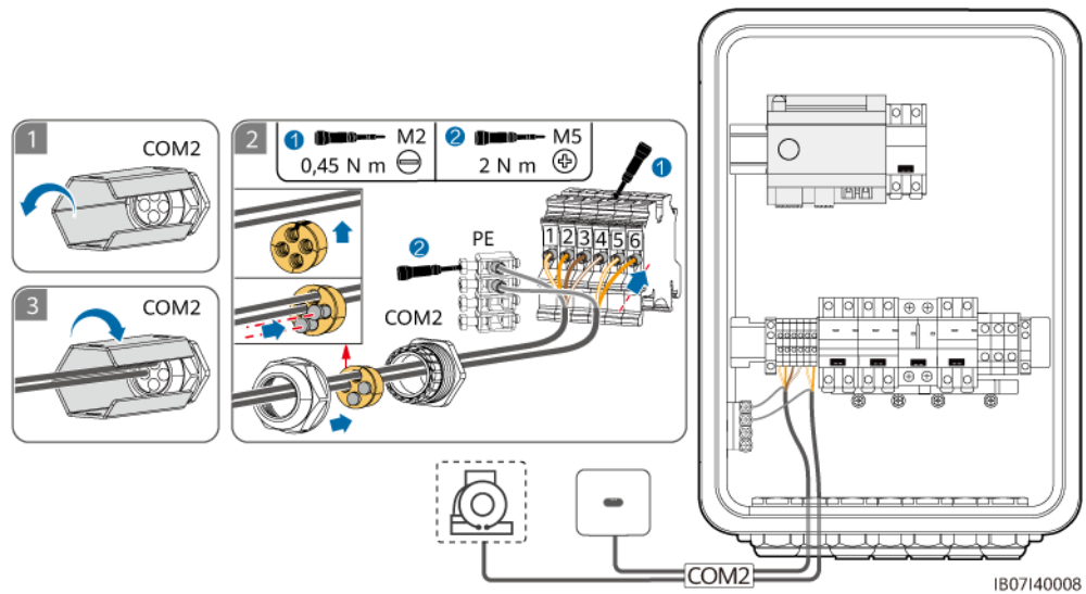
Abbildung 5-26 Anschließen des Signalkabels des SmartGuard (das gestrichelte Kästchen zeigt eine optionale Komponente an)
