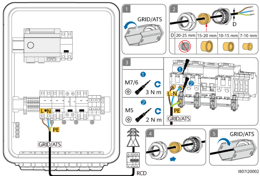
Abbildung 5-11 Anschließen des Netz-AC-Ausgangsstromkabels (L/N Single-Live-Kabelverbindung)
