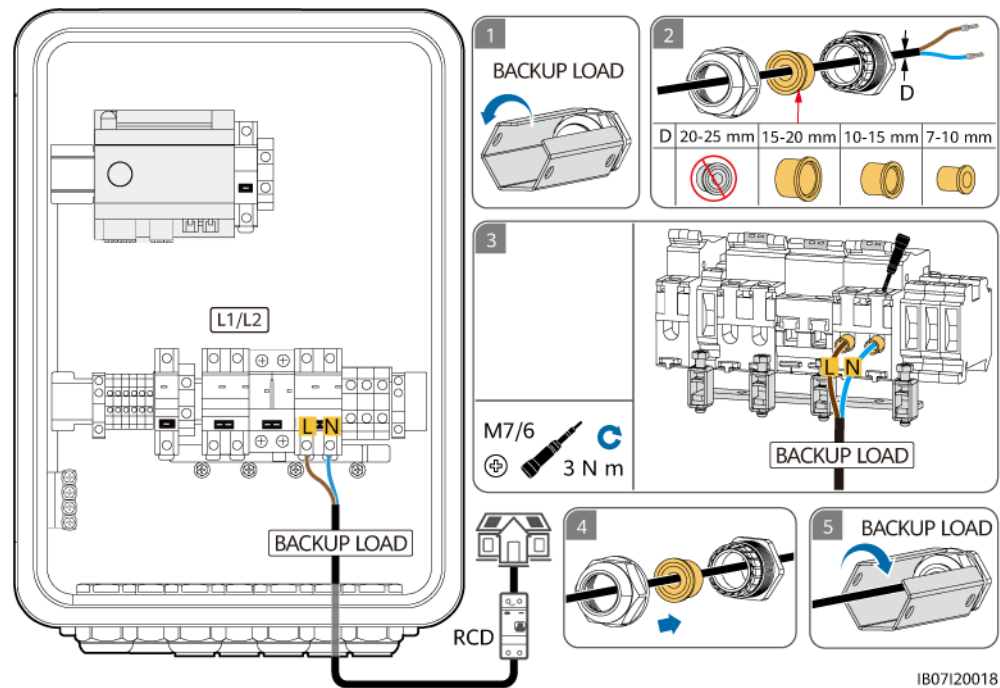
Abbildung 5-20 Anschließen des Ausgangstromkabels der Backup-Last der SmartGuard-63A-AUS0
