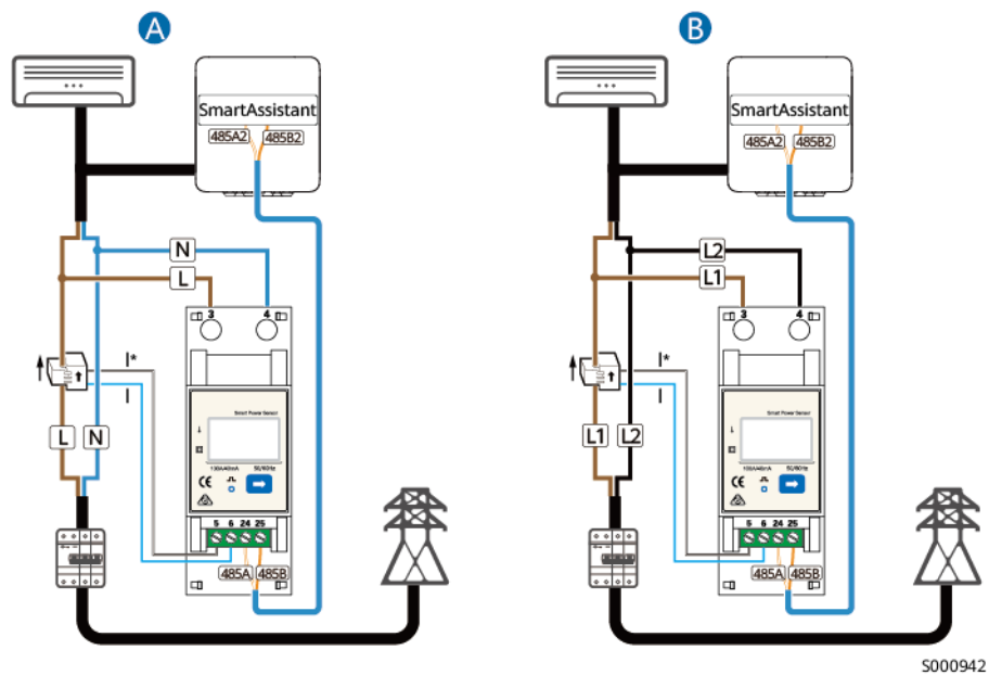
Abbildung 5-30 Anschließen des Kommunikationskabels des Stromzählers
