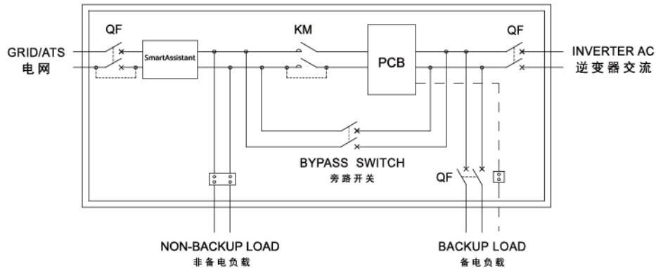
Abbildung 2-11 Elektrischer Schaltplan des SmartGuard
