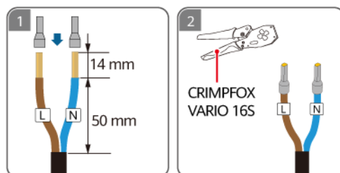
Abbildung 5-18 Crimpen der AC-Kabelendverschlüsse des SmartGuard-63A-AUS0
