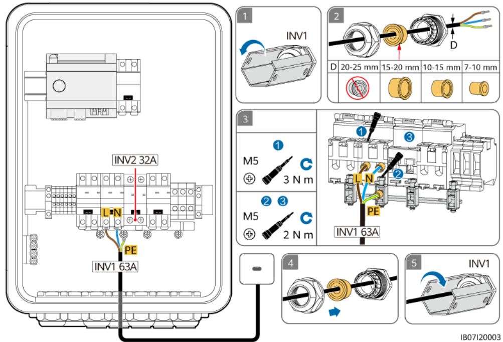
Abbildung 5-15 Anschließen des AC-Eingangsstromkabels vom Wechselrichter (L/N Single-Live-Kabelverbindung)
