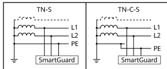
Abbildung 2-8 Erdungssystem (L1/L2 Dual-Live-Kabelverbindung)
