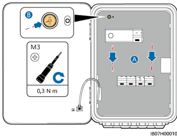
Abbildung 6-1 Schließen des Deckels
