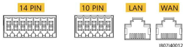
Abbildung 5-27 Anschlussdefinitionen
