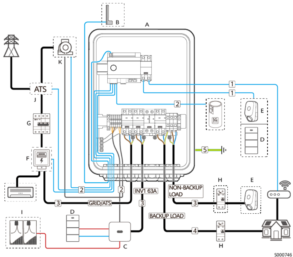
Abbildung 5-1 Kabelverbindungen (gestrichelte Kästchen stehen für optionale Konfigurationen)
