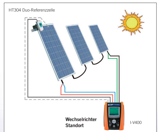
Anschluss I-V400 direkt an HT304
